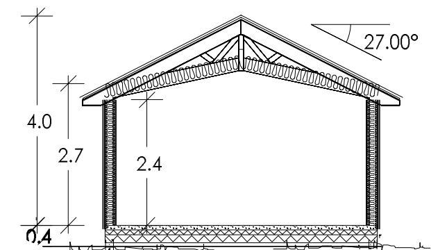
Snitt B-B
