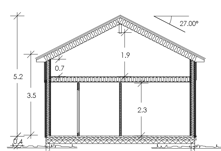
Snitt A-A
